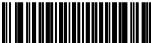
Enable Code 93
